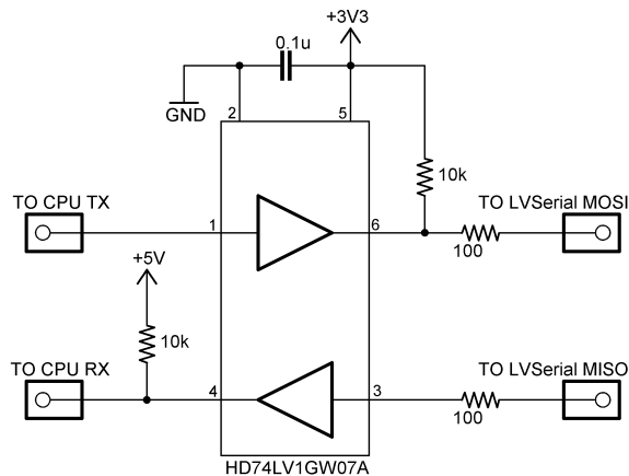
図 2 TTL レベルのコントローラとの接続
