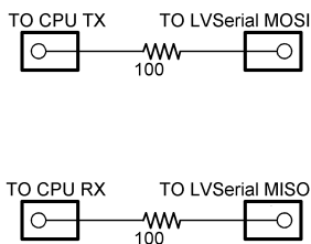
図 1 LVTTTL レベルのコントローラとの接続
